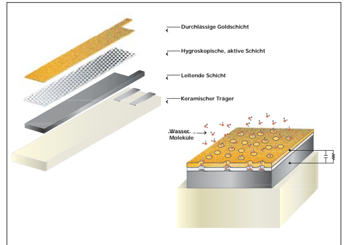
Keramik Metalloxid Sensorschichtaufbau
